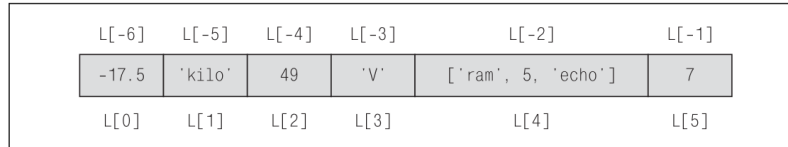
Рис. 2: Позиции элементов в списке
