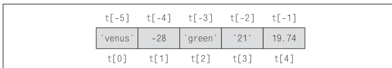
Рис. 1: Позиции элементов в кортеже
